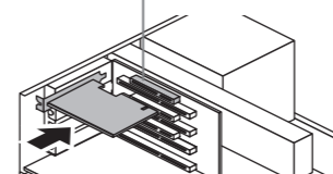
PCIバススロットのコネクタ
